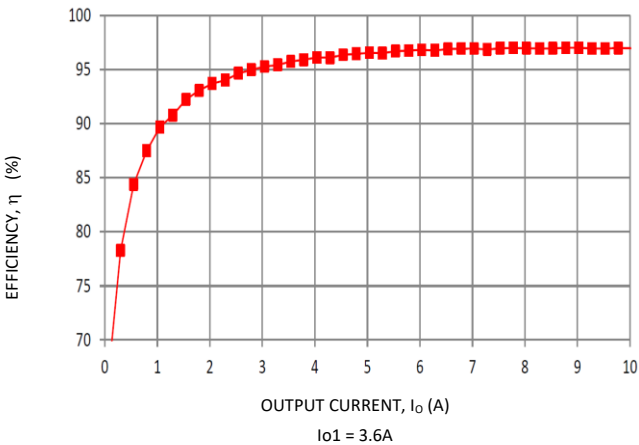
Fig 9a: Efficiency
