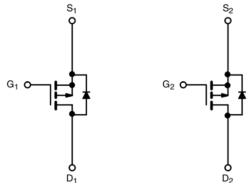
P-Channel MOSFET
